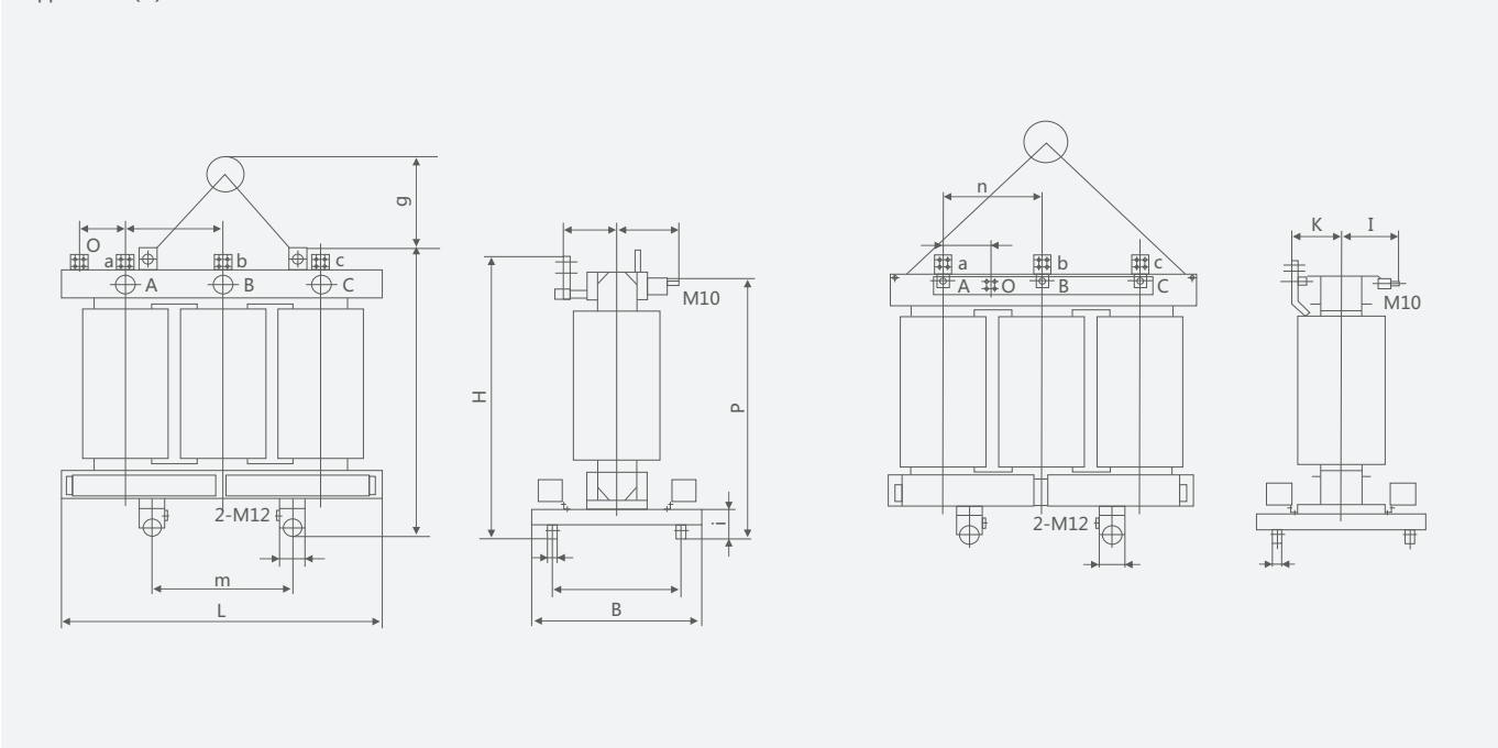
Модели SG(B)10-100 - 400 кВА
