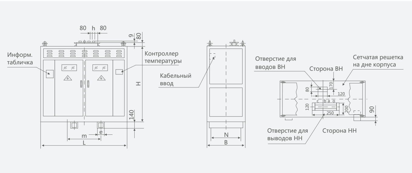
Присоединительные размеры вводов НН
