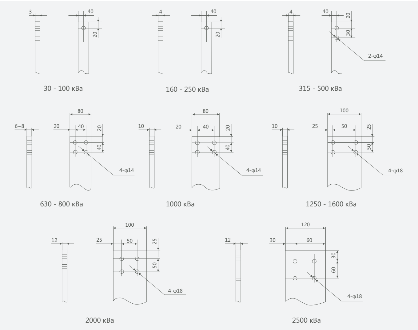
Присоединительные размеры вводов НН
