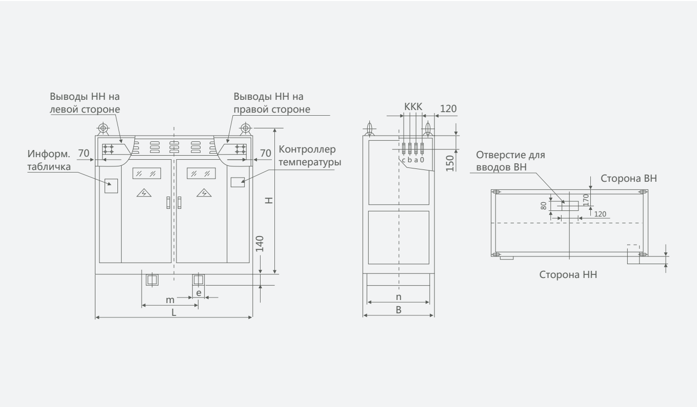
Силовой трансформатор серии SG(B)10
