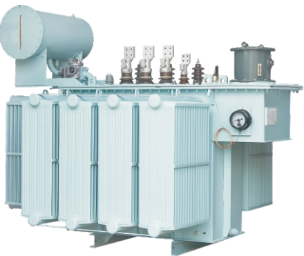
Серии SZ9 (11,13): трансформаторы с переключением под нагрузкой на напряжение 10 кВ
