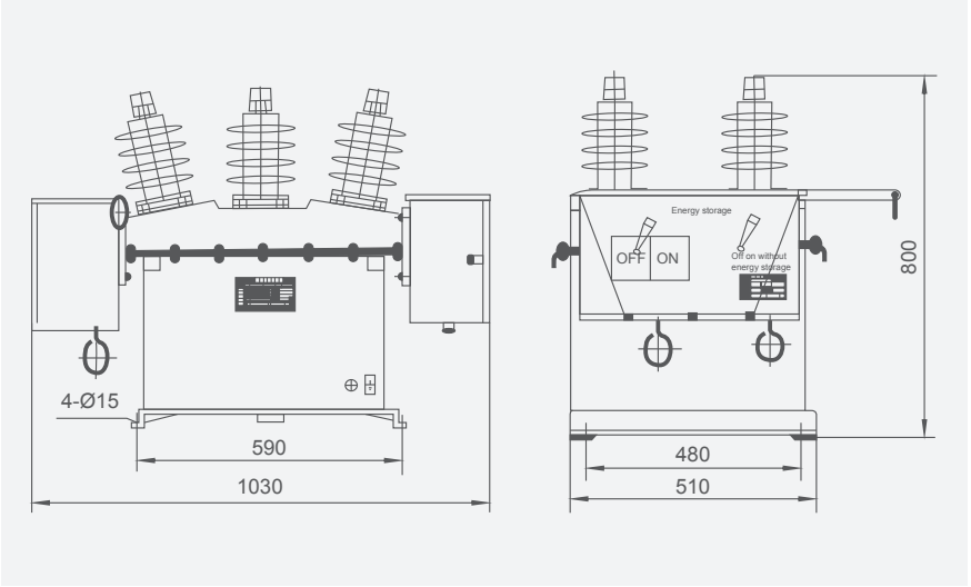
Рисунок 4. Габаритные и монтажные размеры ZW8-12 / electric PT
