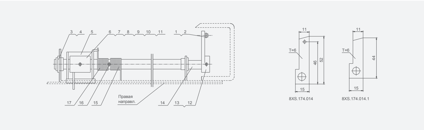
Список компонентов блокирующего устройства для Din-рейки (5XS.363.011)
