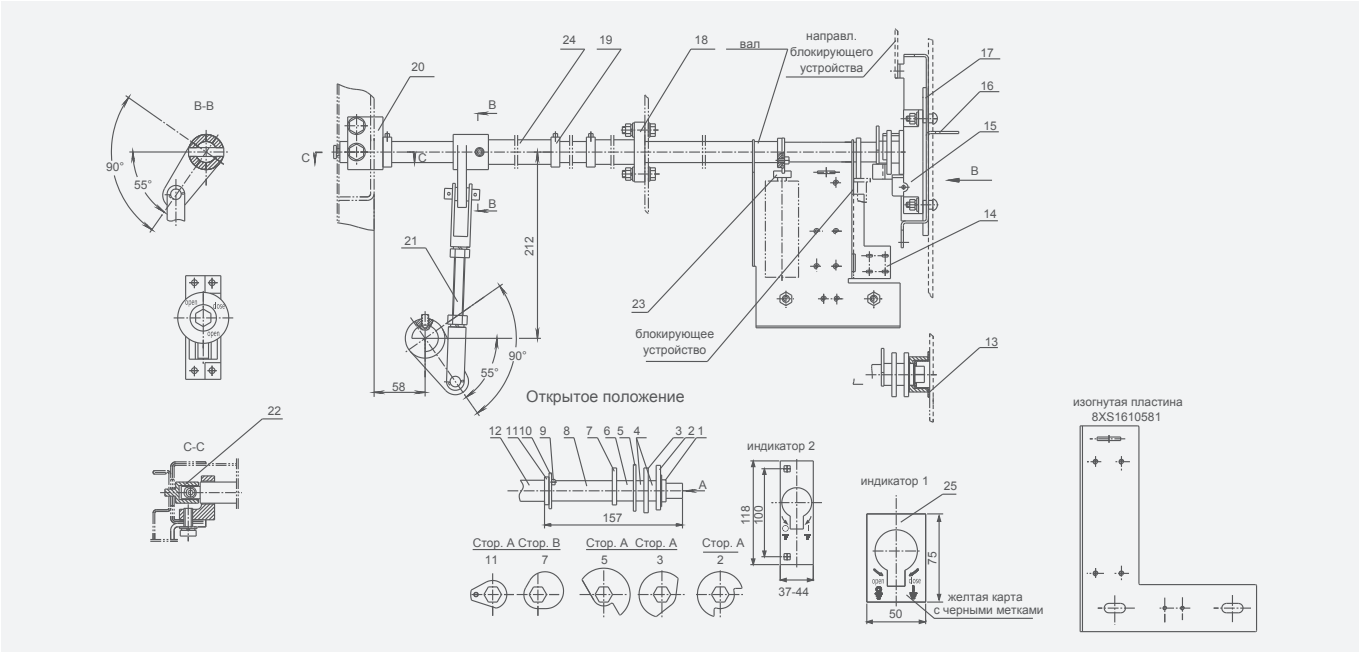
Список компонентов механизма блокировки заземлителя (соединительная тяга) 5XC.363.010
