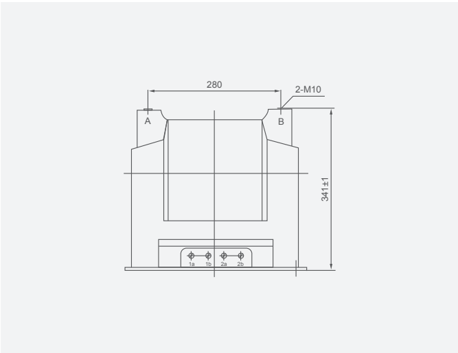
Схема подключения
