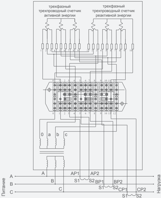
Схема подключения 3 трехфазного четырехпроводного счетчика электроэнергии
