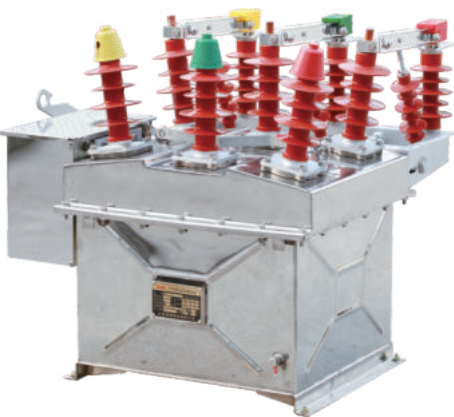
ZW8-12
