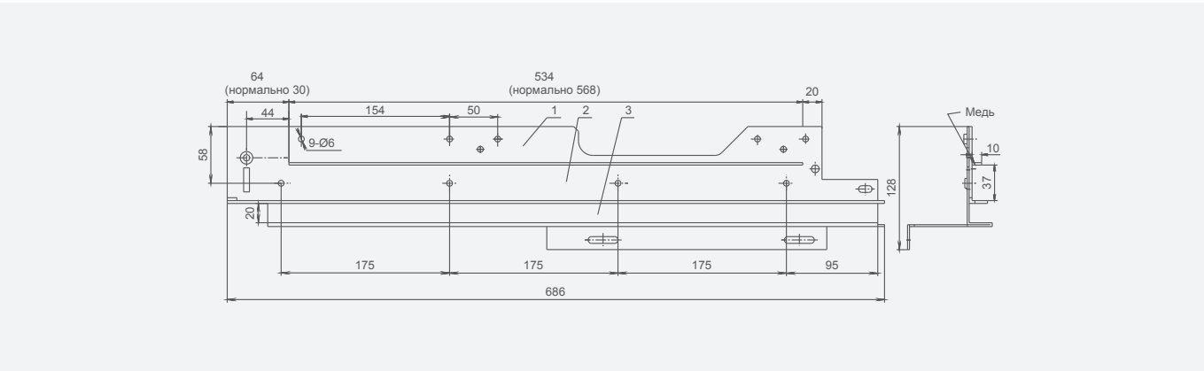
Сборочный чертеж блокирующего устройства для Din-рейки (5XS.363.011)
