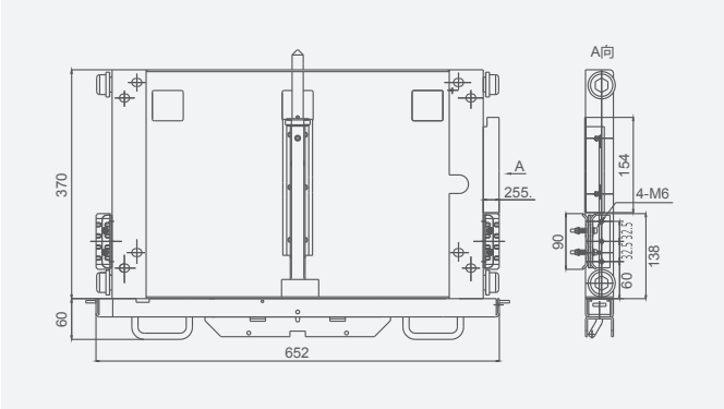
(4) Монтажные размеры заземляющего зажима
