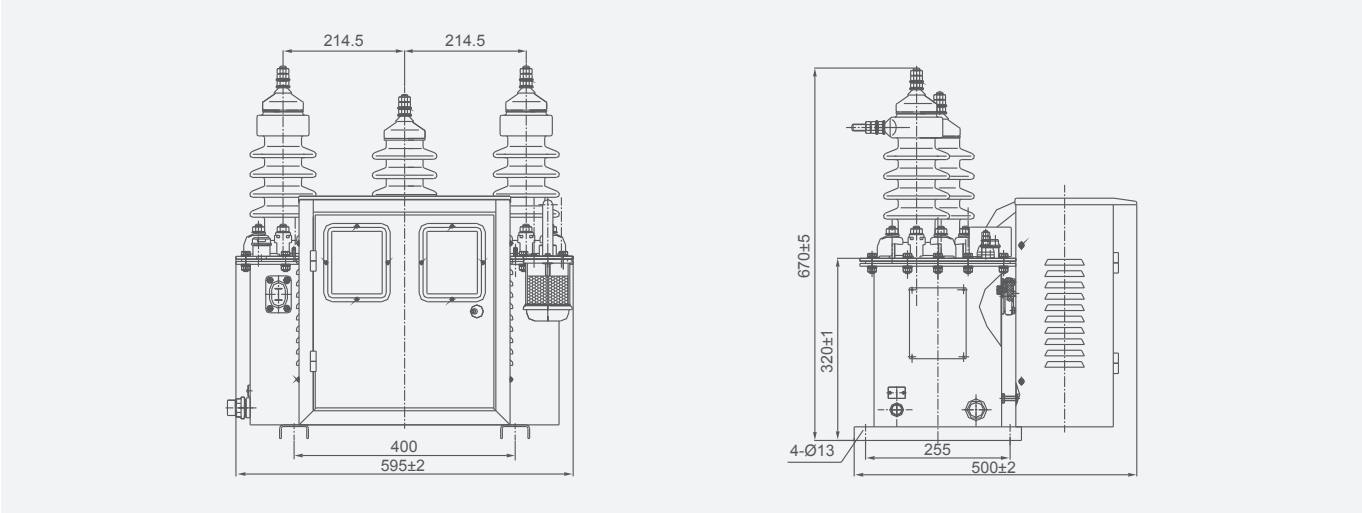
Схема 3: Габаритные и монтажные размеры трехфазного трехпроводного измерителя 35 кВ (трехфазный двухкомпонентный)
