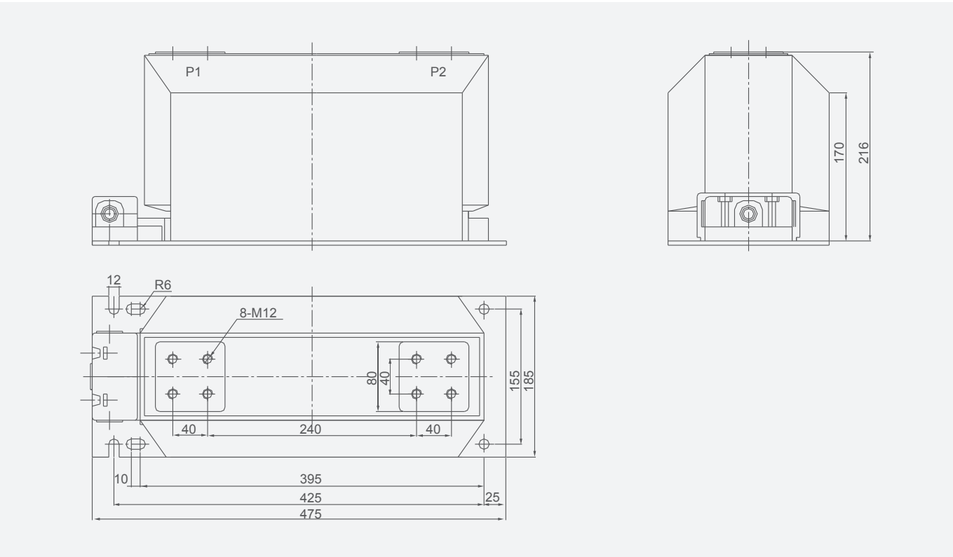
Рис. 6. Габаритные и монтажные размеры трансформатора токаLZZBJ9-10A5G 1200-3000A
