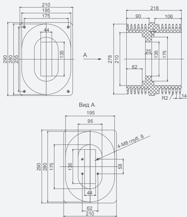
Проходной изолятор 24KV-175*255*218, габаритные и монтажные размеры
