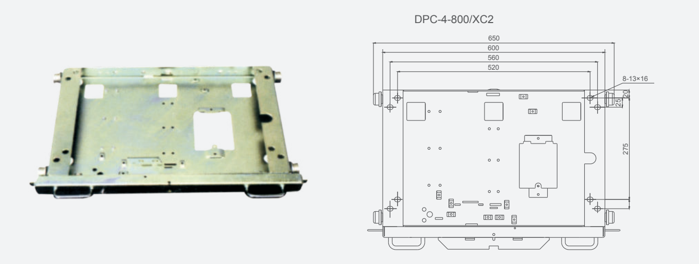
7. DPC-4-800/XC2: габаритные и монтажные размеры
