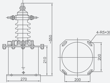
Рис. 2. Габаритные и монтажные размеры для LJWD-10 (с двумя классами)
