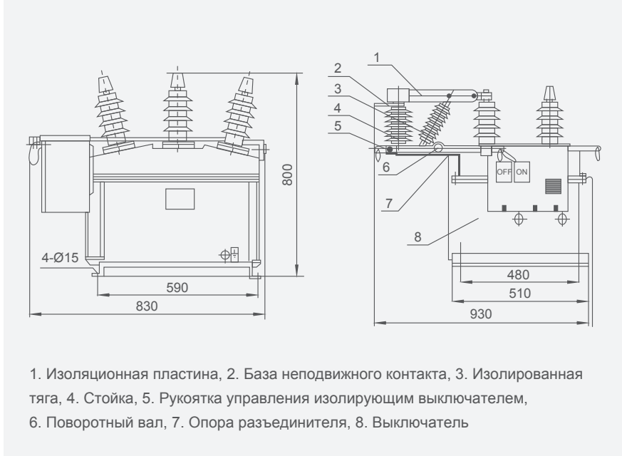
Рисунок 2. Габаритные и монтажные размеры ZW8-12G/Т
