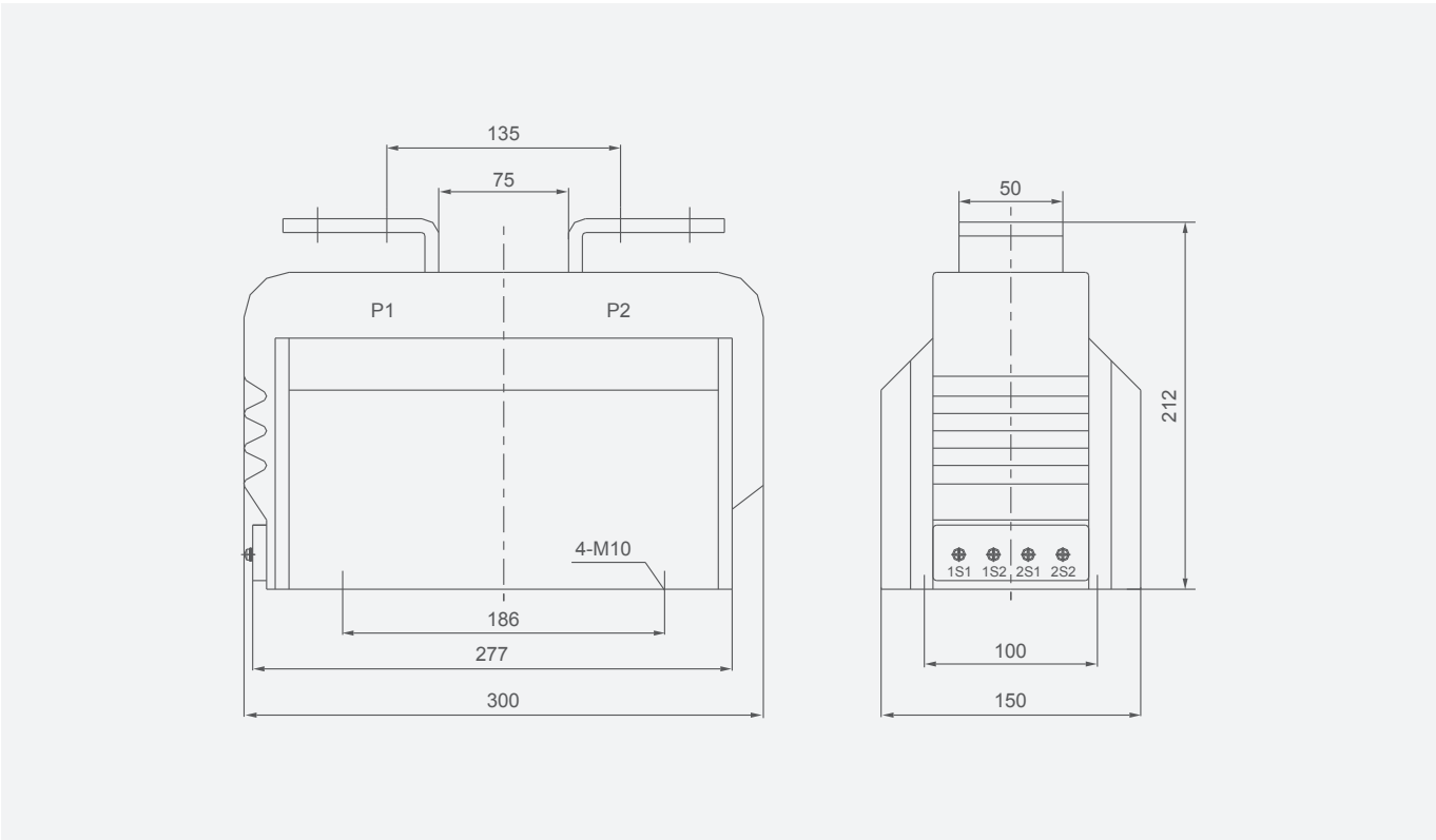
Схема 2. Габаритные и монтажные размеры LFSB-10(LZZBJ-10)
