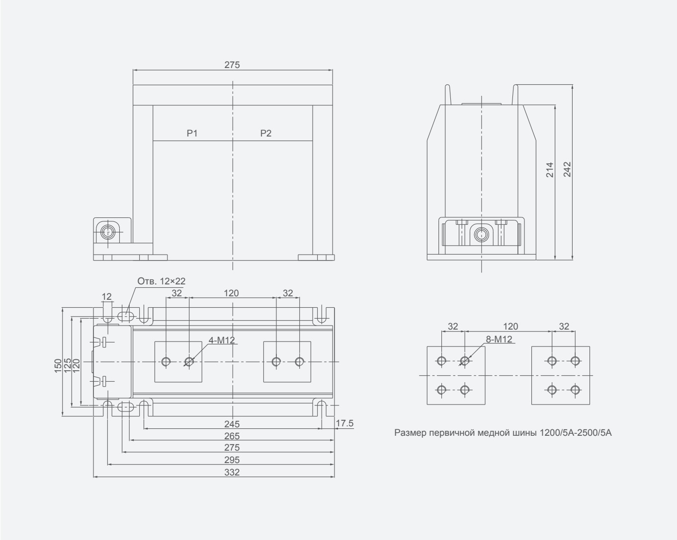
LZZBJ18-10/185h/2 (эквивалент AS12/185h/2S)
