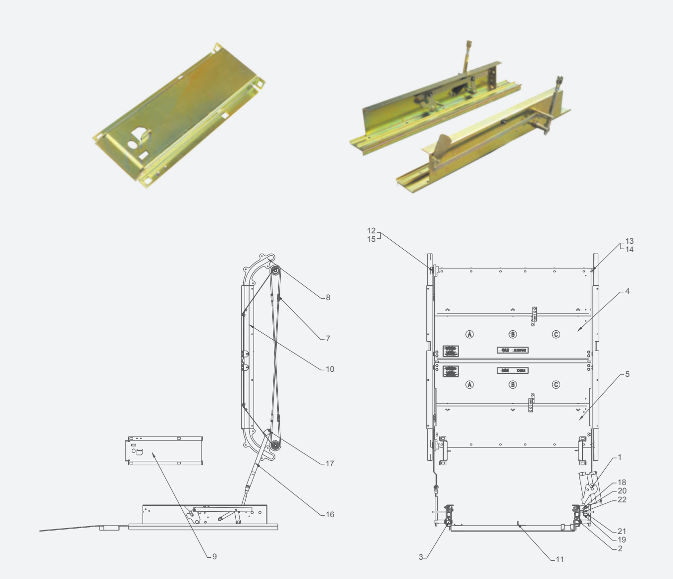
Затворный механизм KYN61C
