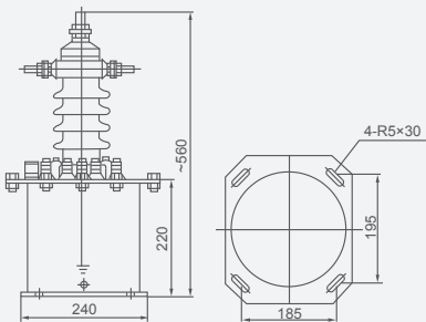
Рис. 1. Габаритные и монтажные размеры для LJW-10 (с одним классом)
