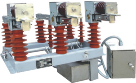
FZW32-12(40.5)
