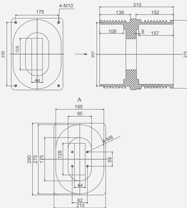
Проходной изолятор 24KV-175*255*310, габаритные и монтажные размеры
