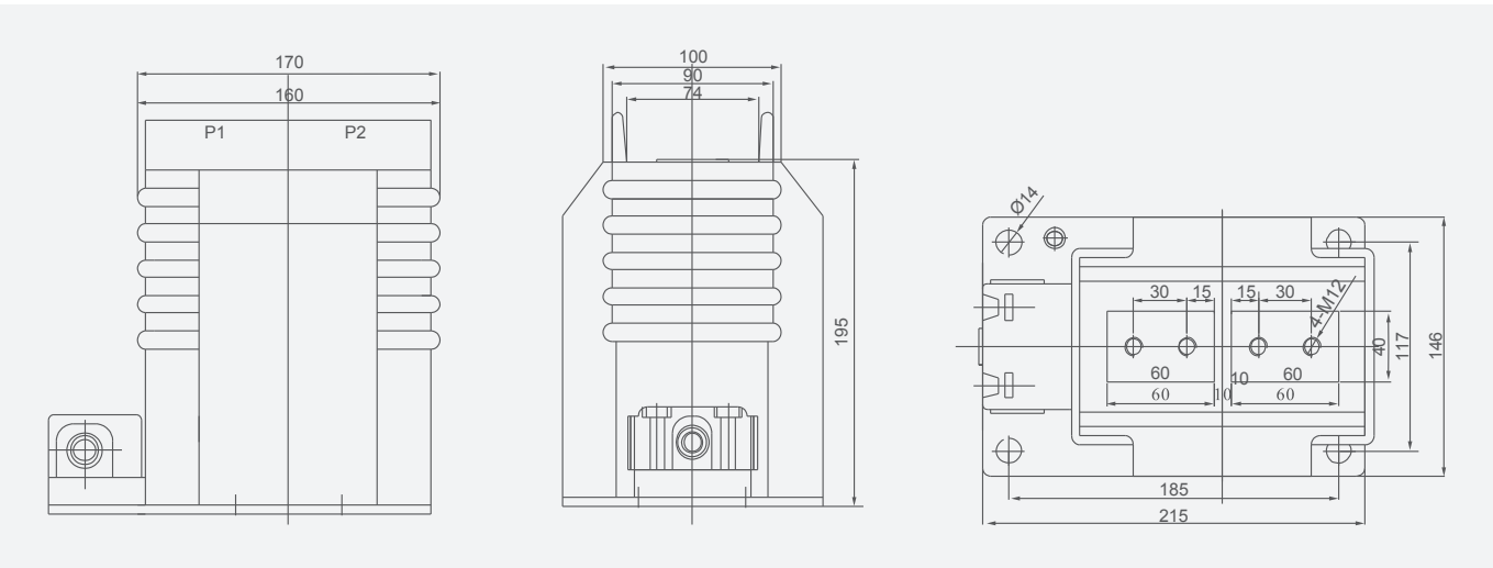
LZZBJ18-10 взаимная индуктивность, с одной обмоткой
