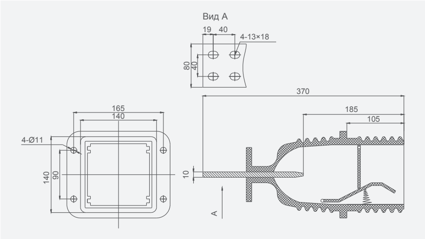
Проходной изолятор 10KV-100*100, габаритные и монтажные размеры
