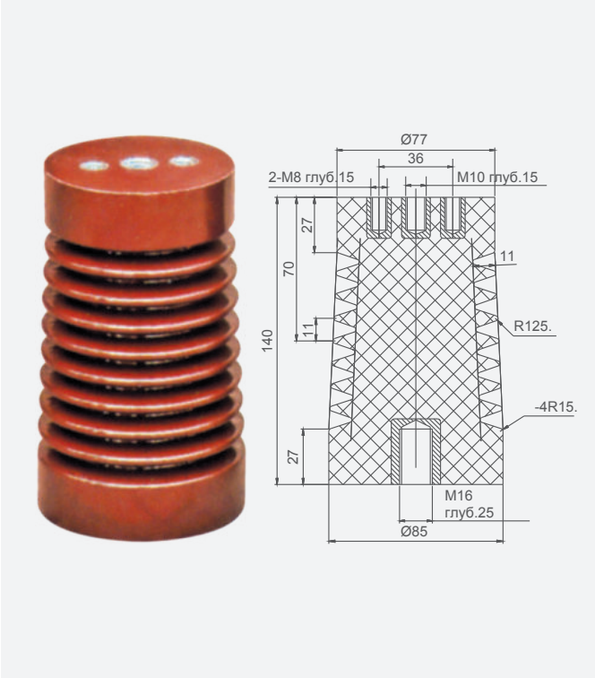
Изделие: высоковольтный изолятор Модель: ZJ-10Q/Ø85×140
