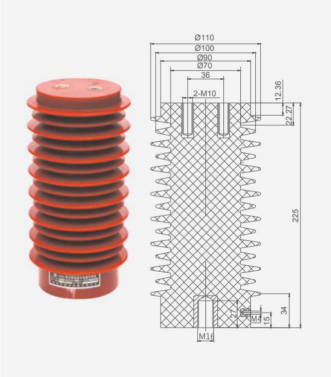
Изделие: датчик Модель: CG102-24Q/Ø110×225
