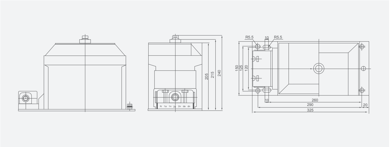
Рис. 1. Габаритные и монтажные размеры JDZ(F)18-6,10B
