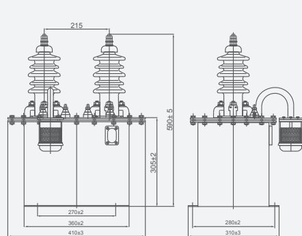
Рис. 3. Габаритные и монтажные размеры для LJW(D)-10
