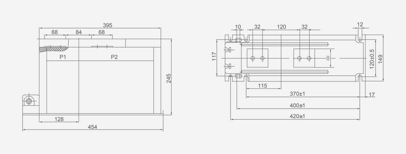
LZZBJ18-10/185h/4 (эквивалент AS12/185h/4S)
