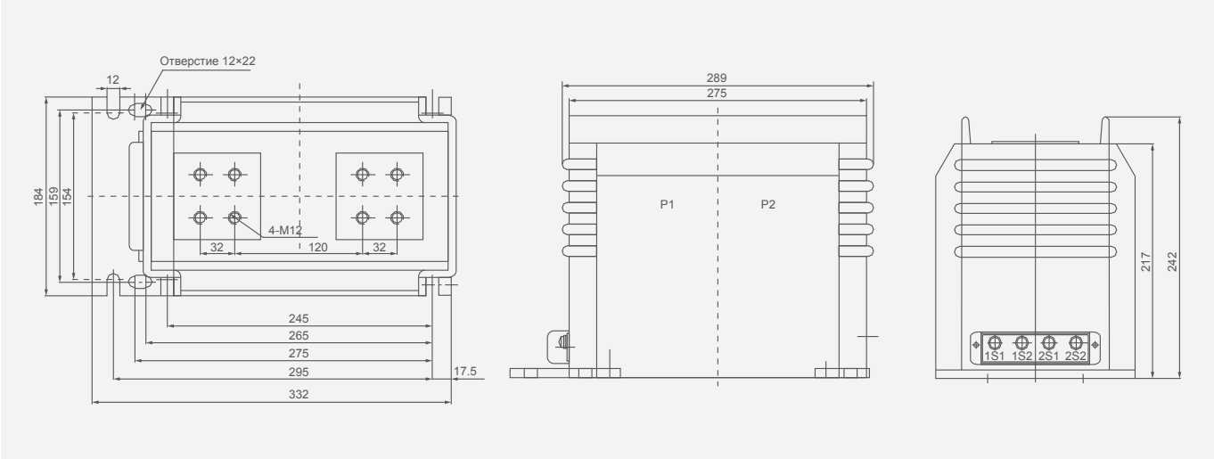
LZZBJ18-10/185h/2 (эквивалент AS12/185h/2S)
