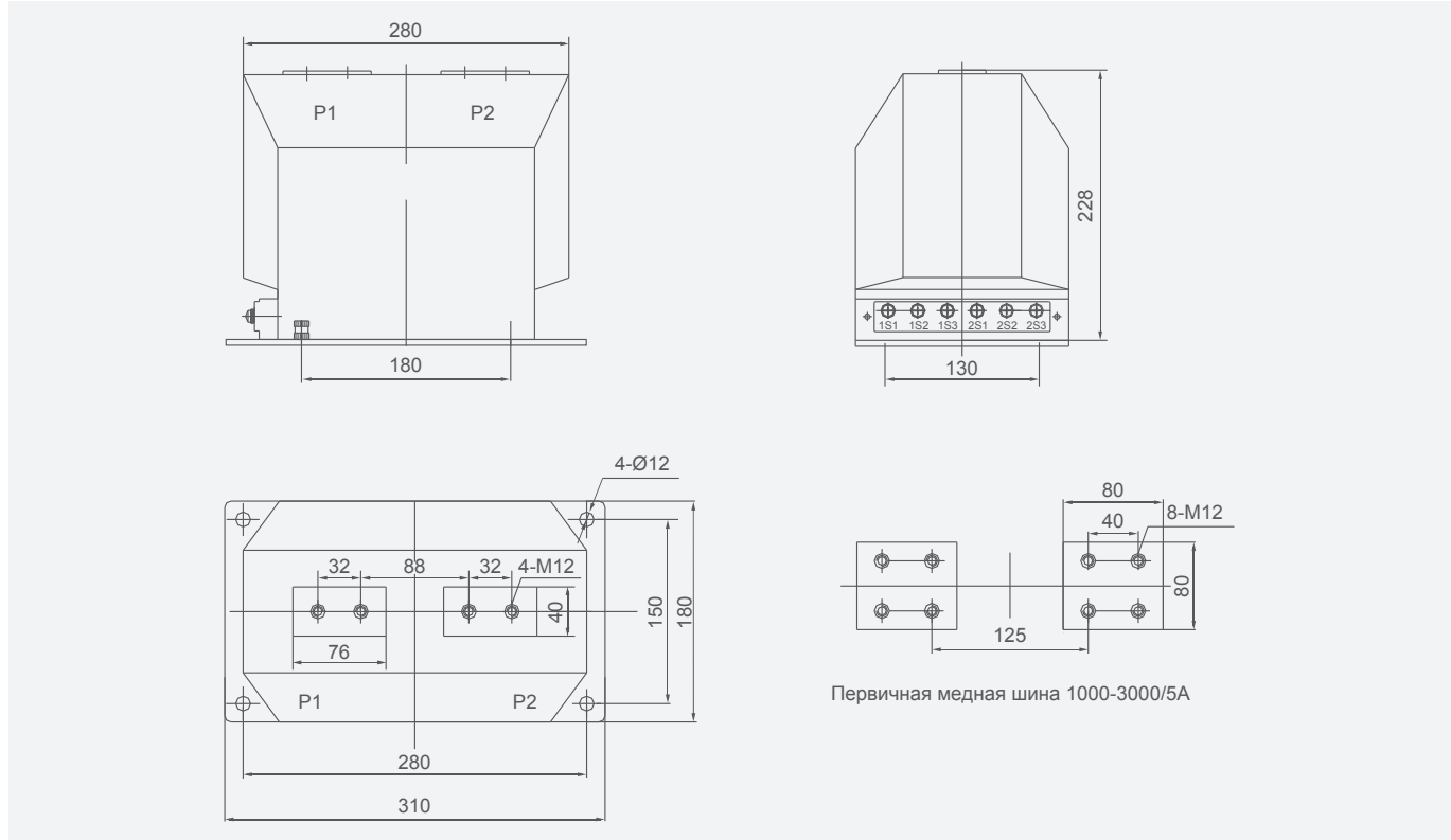
Рис 4. Габаритные и монтажные размеры трансформатора тока LZZBJ9-10C 2
