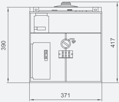
Выключатель нагрузки, вид спереди
