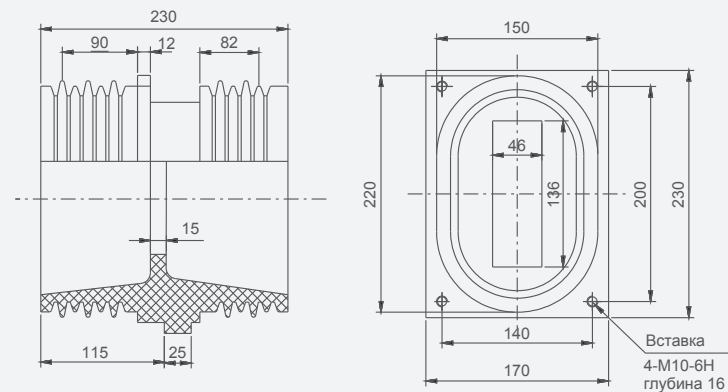
Проходной изолятор TG3-10Q/170×230, габаритные и монтажные размеры
