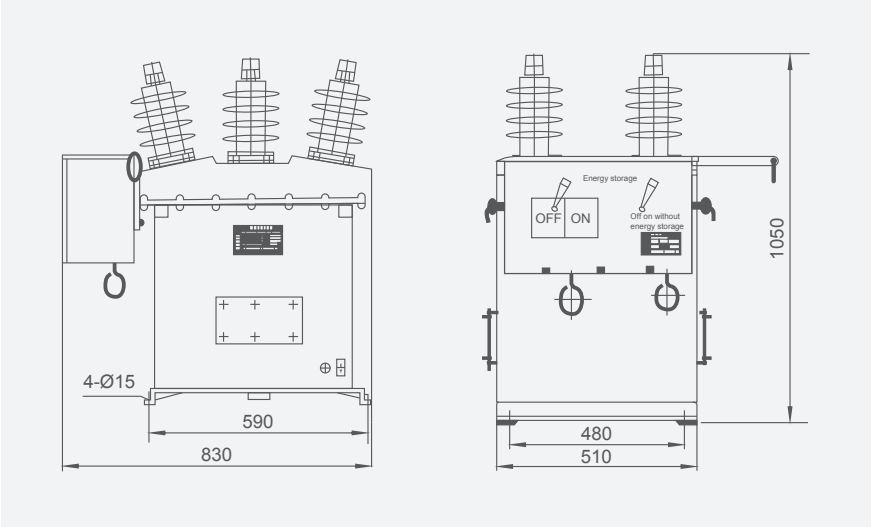
Рисунок 3. Габаритные и монтажные размеры ZW8-12/C, ZW28-12/PT
