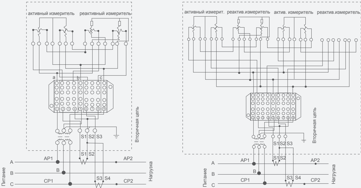
Трехфазная трехпроводная одиночная измерительная схема 1 Трехфазная трехпроводная двойная измерительная схема 2
