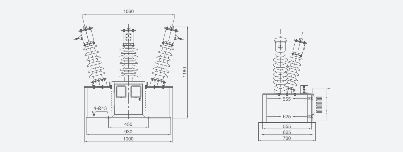
Схема 4: Габаритные и монтажные размеры трехфазного четырехпроводного измерителя 35 кВ (трехфазный трехкомпонентный)
