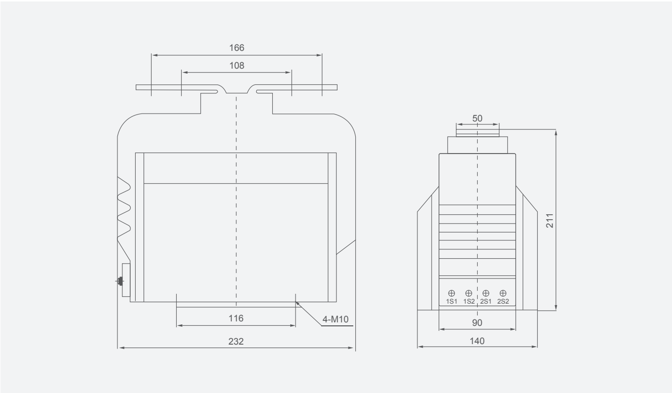
Схема 1. Габаритные и монтажные размеры LFS-10Q(LZZB-10)
