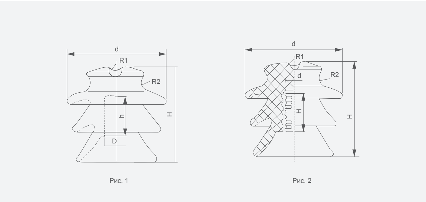
Габаритные размеры и артикулы
