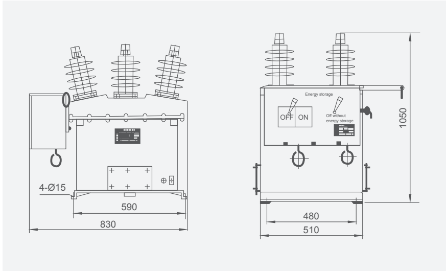
Рисунок 1. Габаритные и монтажные размеры ZW8-12/Т
