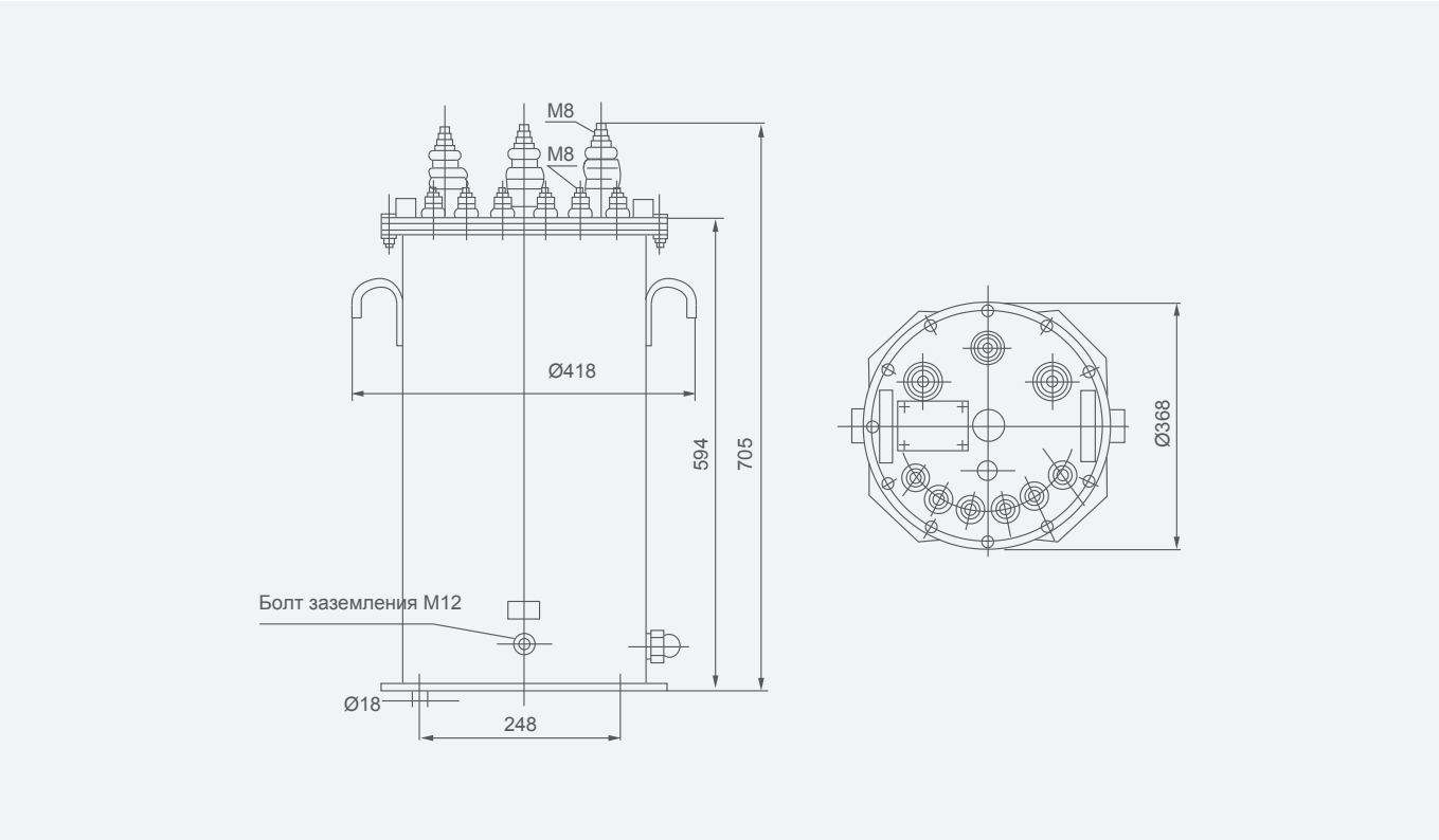
Рис. 1. Габаритные и монтажные размеры для JSJW-6
