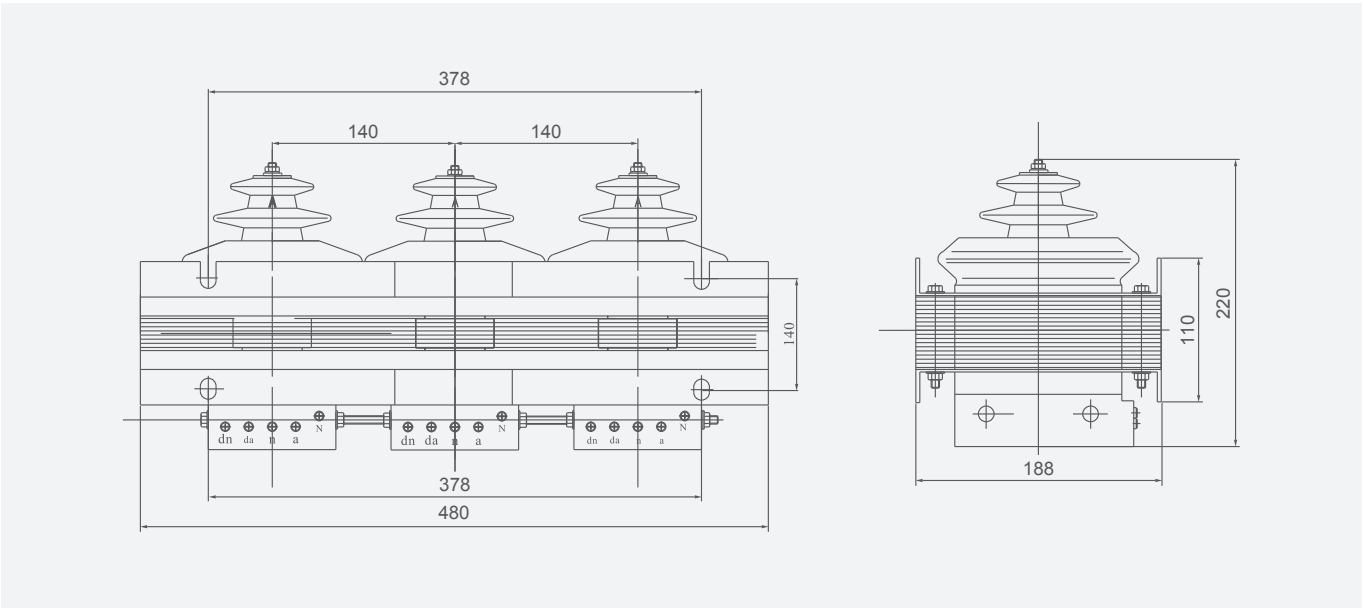
JSZW-3,6,10 кВ
