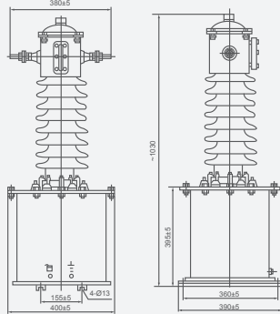
Рис. 4. Габаритные и монтажные размеры для LJW(D)-35
