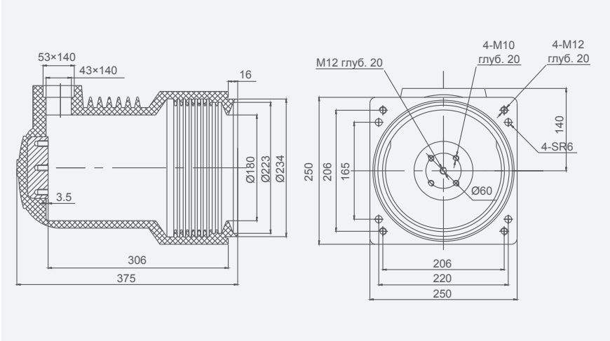
Соединительная коробка СНЗ-24KV-252 (номинальный ток ≤ 3150-4000А), габаритные и монтажные размеры
