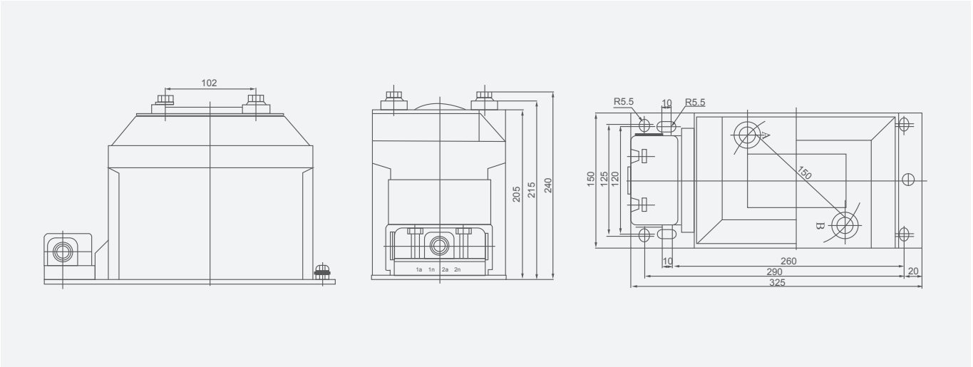
Рис. 3. Габаритные и монтажные размеры JDZX10-6,10(REL10)
