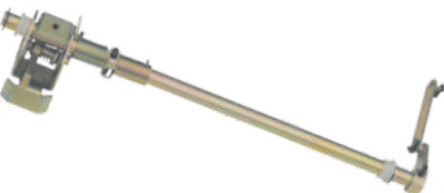
Блокирующее устройство для DIN-рейки 5XS.363.011
