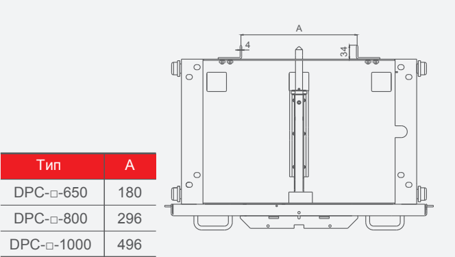
(3) Монтаж заземляющего контакта
