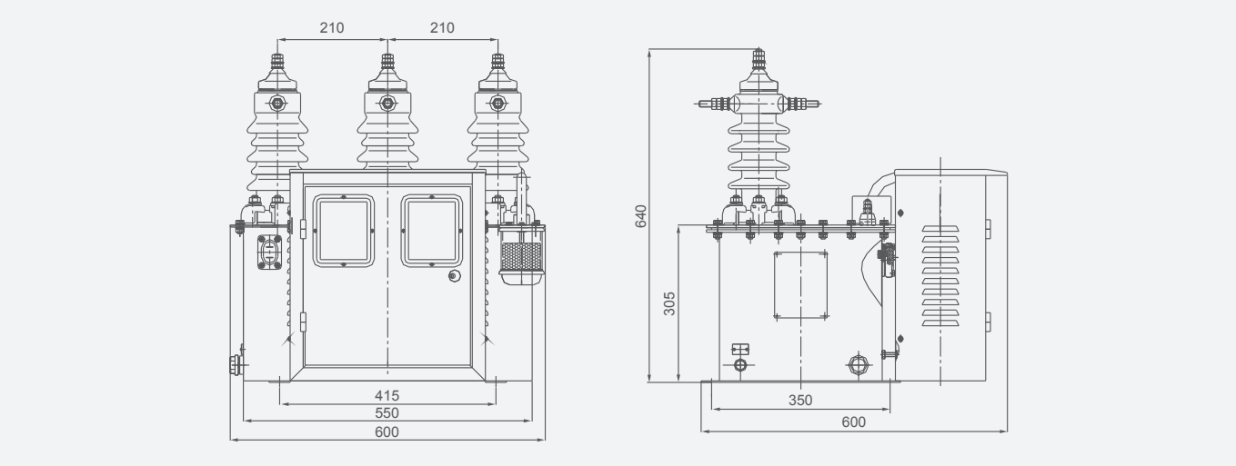
Схема 1: Габаритные размеры и монтажные размеры трехфазного четырехпроводного измерителя 6 кВ, 10 кВ (трехфазный трехкомпонентный)
