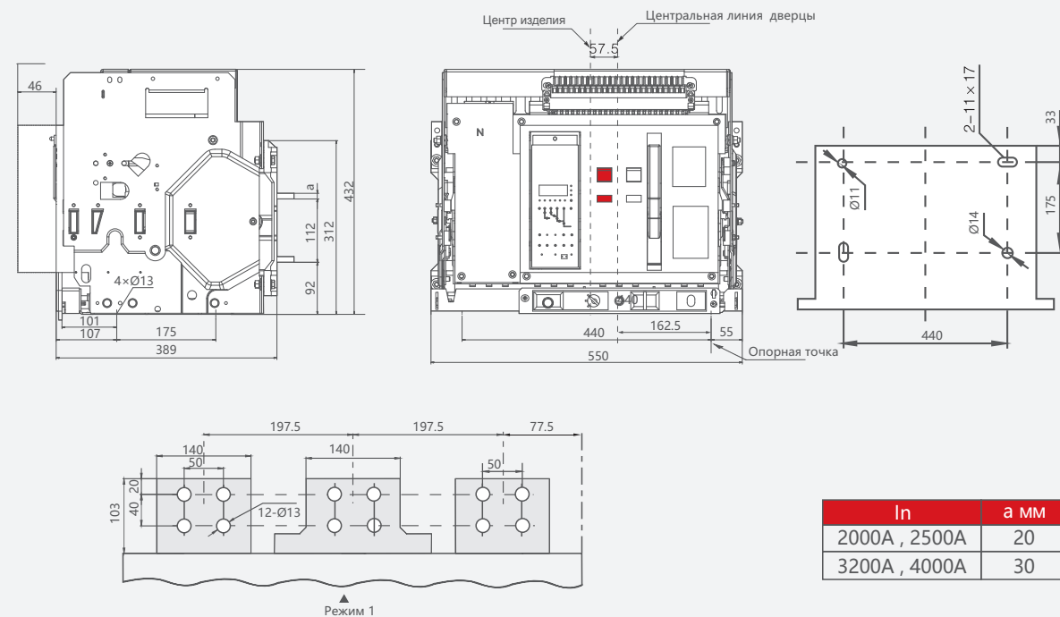
Монтажные и габаритные размеры выкатного выключателя (Imn = 4000А, 3 полюса)
