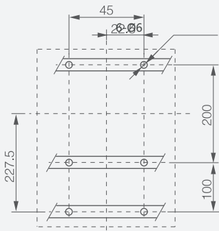
3P: монтаж на направляющие
