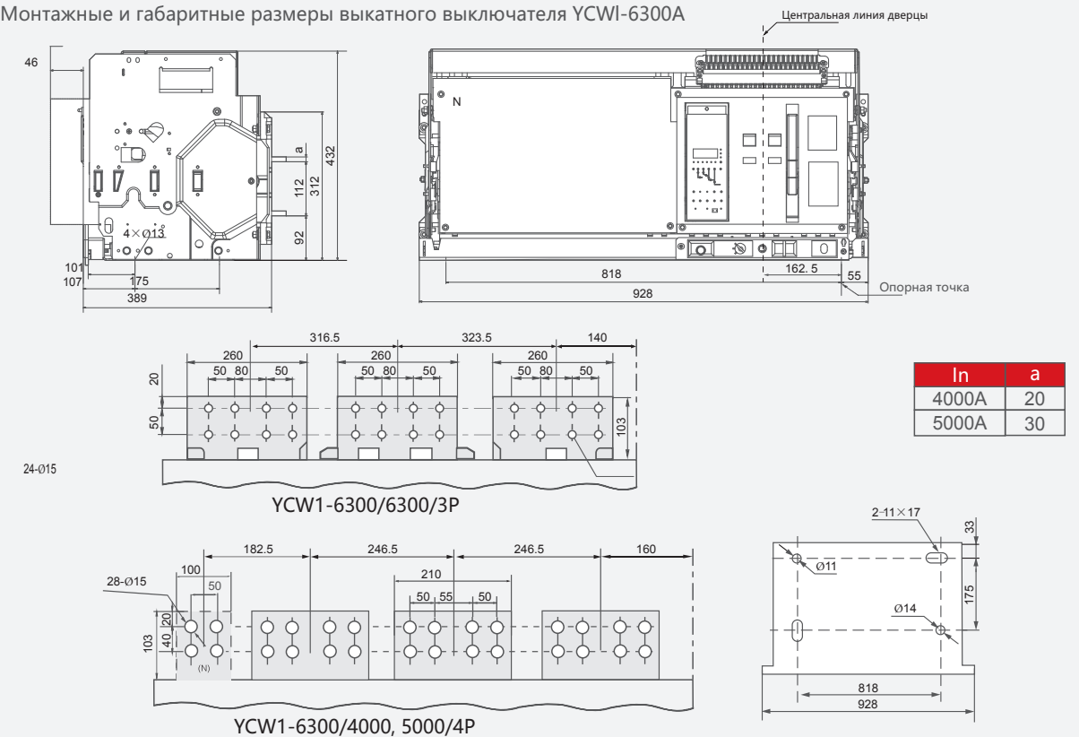
Монтажные и габаритные размеры выкатного выключателя (Inm=6300A) (4000A, 5000A 3P и 4P, как и 6300A 3P)
