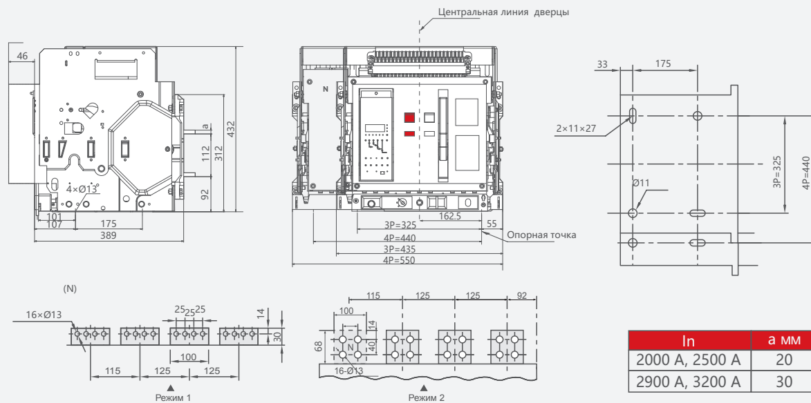
Монтажные и габаритные размеры выкатного выключателя ( I_{nm} = 3200 \text{ A} , 3P, 4P)
